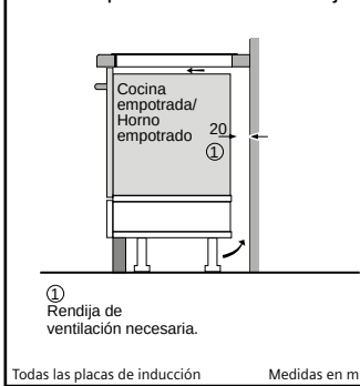
Todas las placas de inducción Medidas en mm
