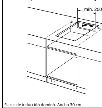
Placas de inducción dominó. Ancho 30 cm Medidas en mm
