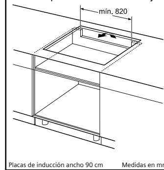
Placas de inducción ancho 90 cm Medidas en mm
