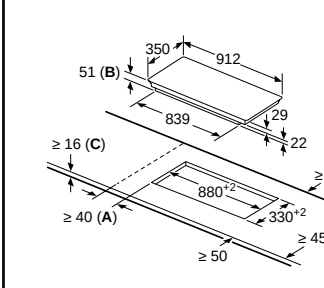
Todas las placas de inducción Medidas en mm
