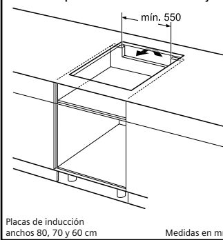
Placas de inducción anchos 80, 70 y 60 cm Medidas en mm
