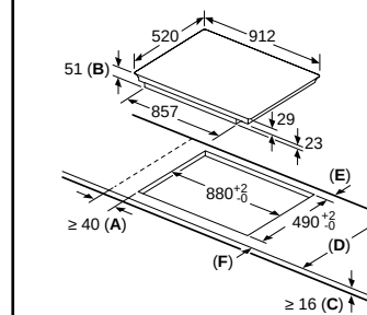
Placas de inducción ancho 90 cm Medidas en mm
